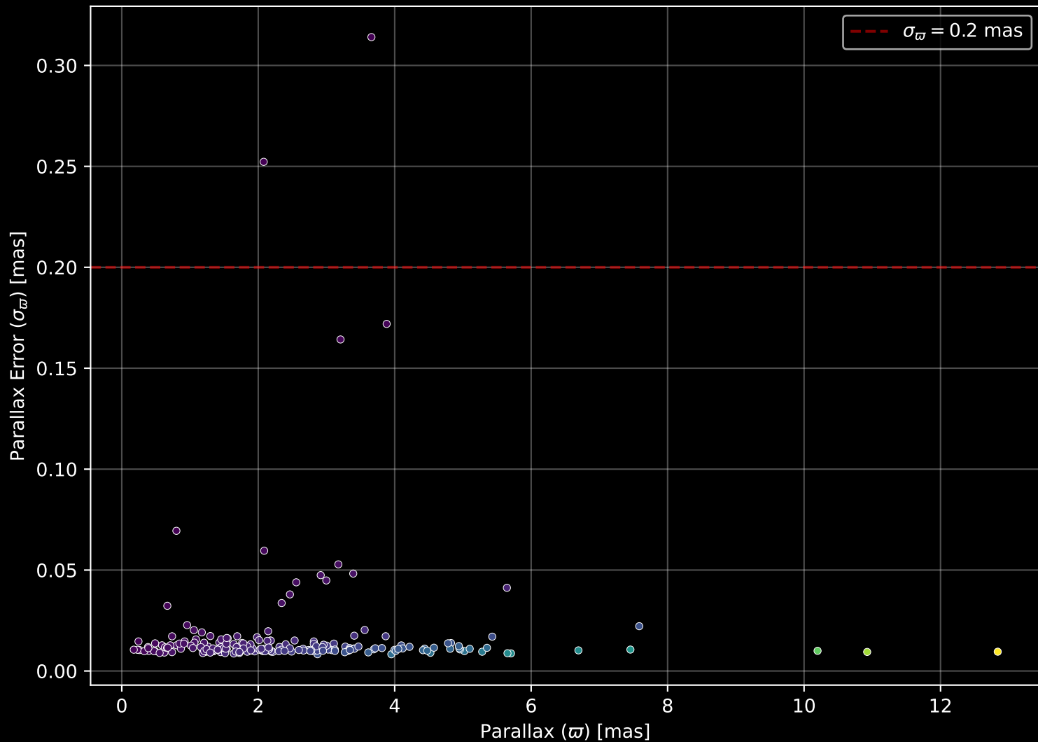
GALAH DR4 Field: [7185] Parallax Quality (n= 213)
