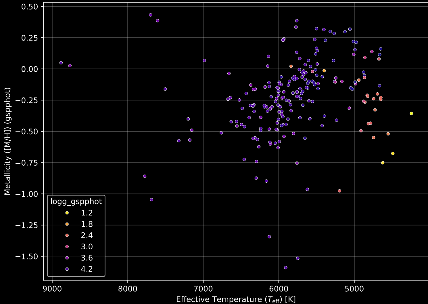
GALAH DR4 Field: [7185] Stellar Population Parameters (n= 213)
