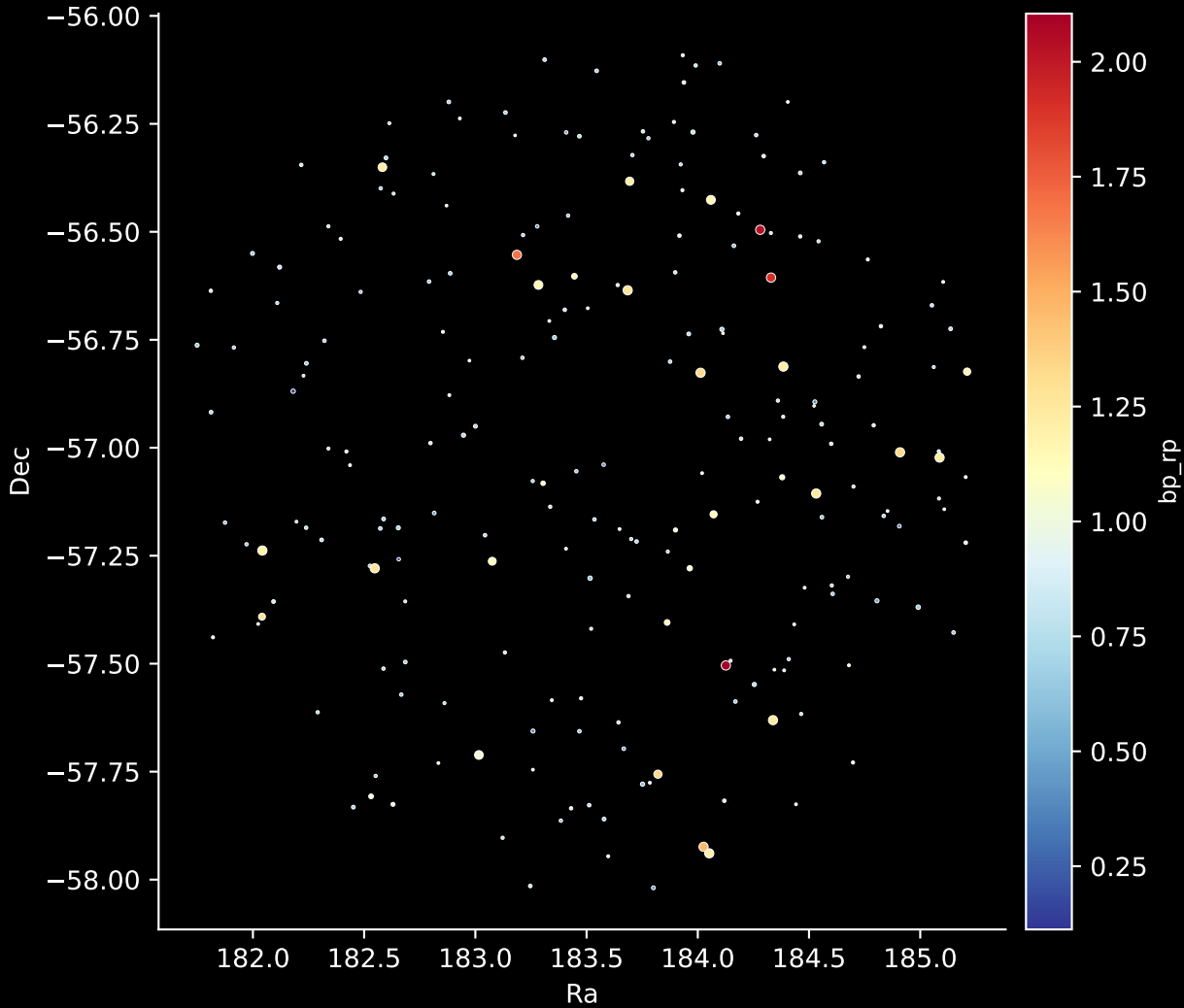
GALAH DR4 Field: [7185] Stars: 213
