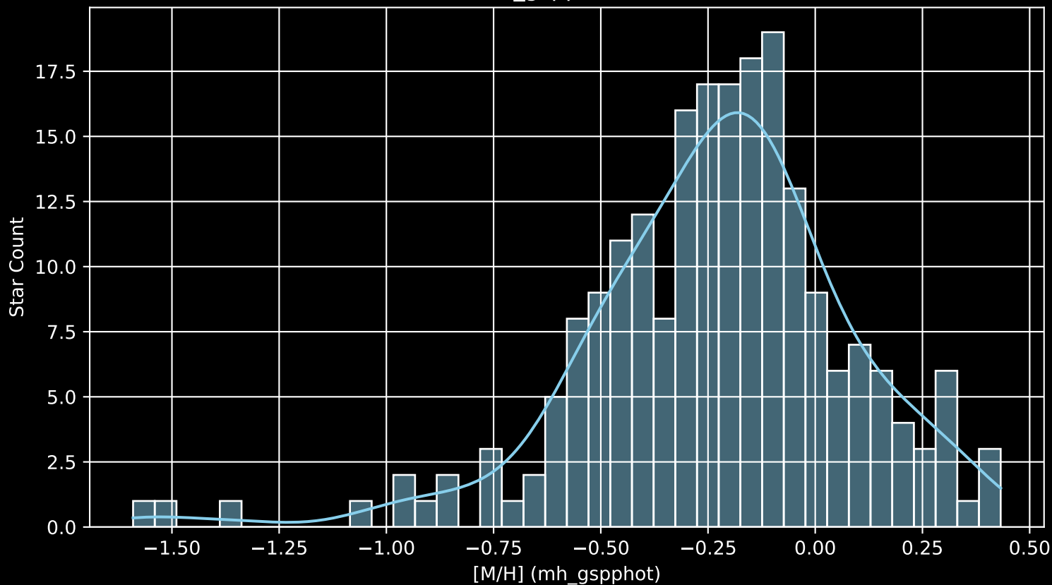
GALAH DR4 Field: [7185] [M/H] (mh_gspphot) (n= 213)
